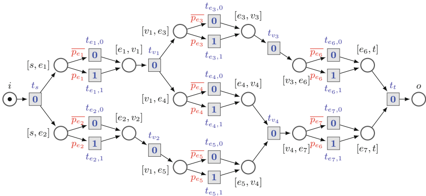
(d) Timed probabilistic workflow net \mathcal{W}_{\mathbf{PN}} .
